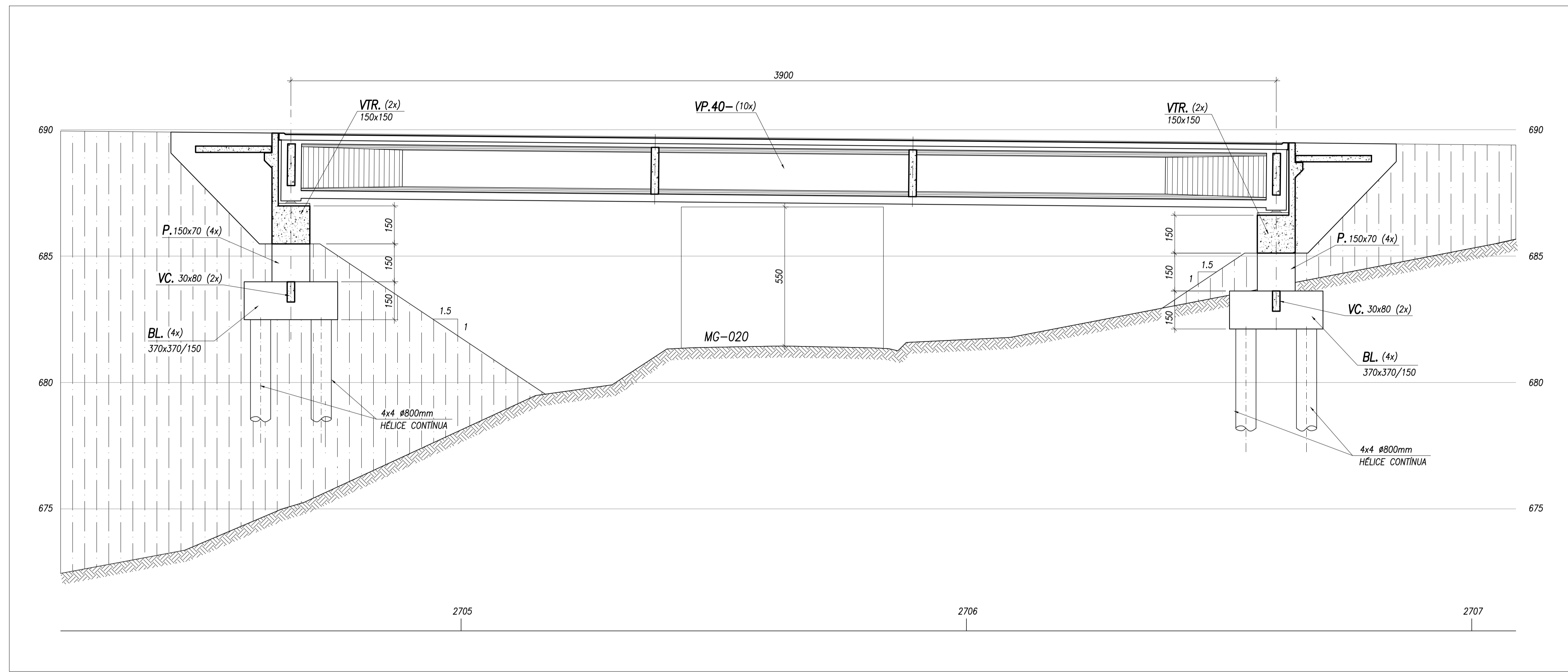
SEÇÃO LONGITUDINAL ESCALA 1:100
