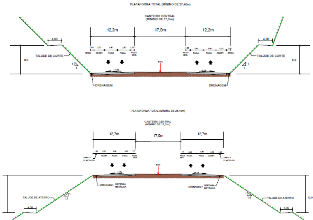
Figura 7: Seção transversal tipo do projeto
