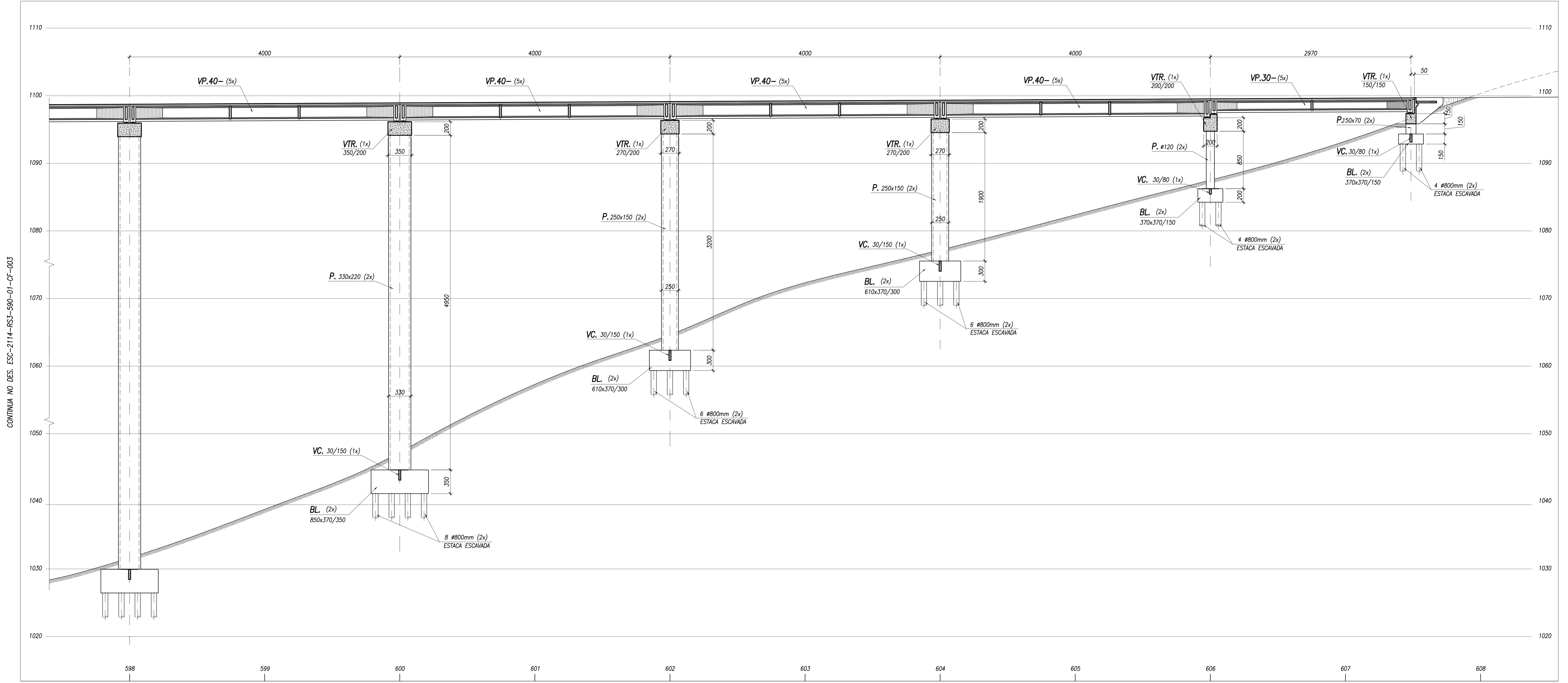
PERFIL LONGITUDINAL - 2a. PARTE ESCALA 1:250
