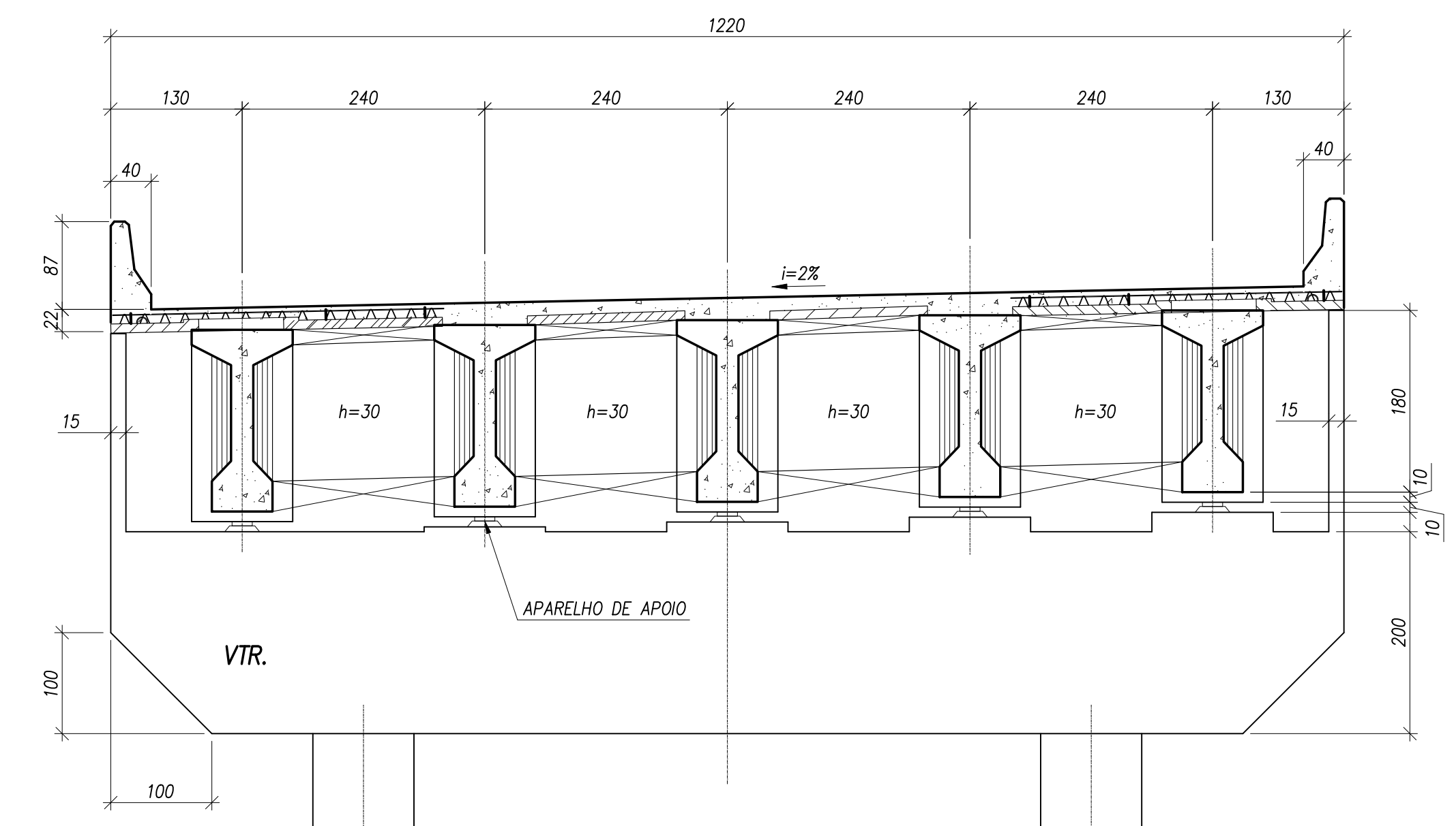
SEÇÃO TRANSVERSAL - APOIO ESCALA 1:50
