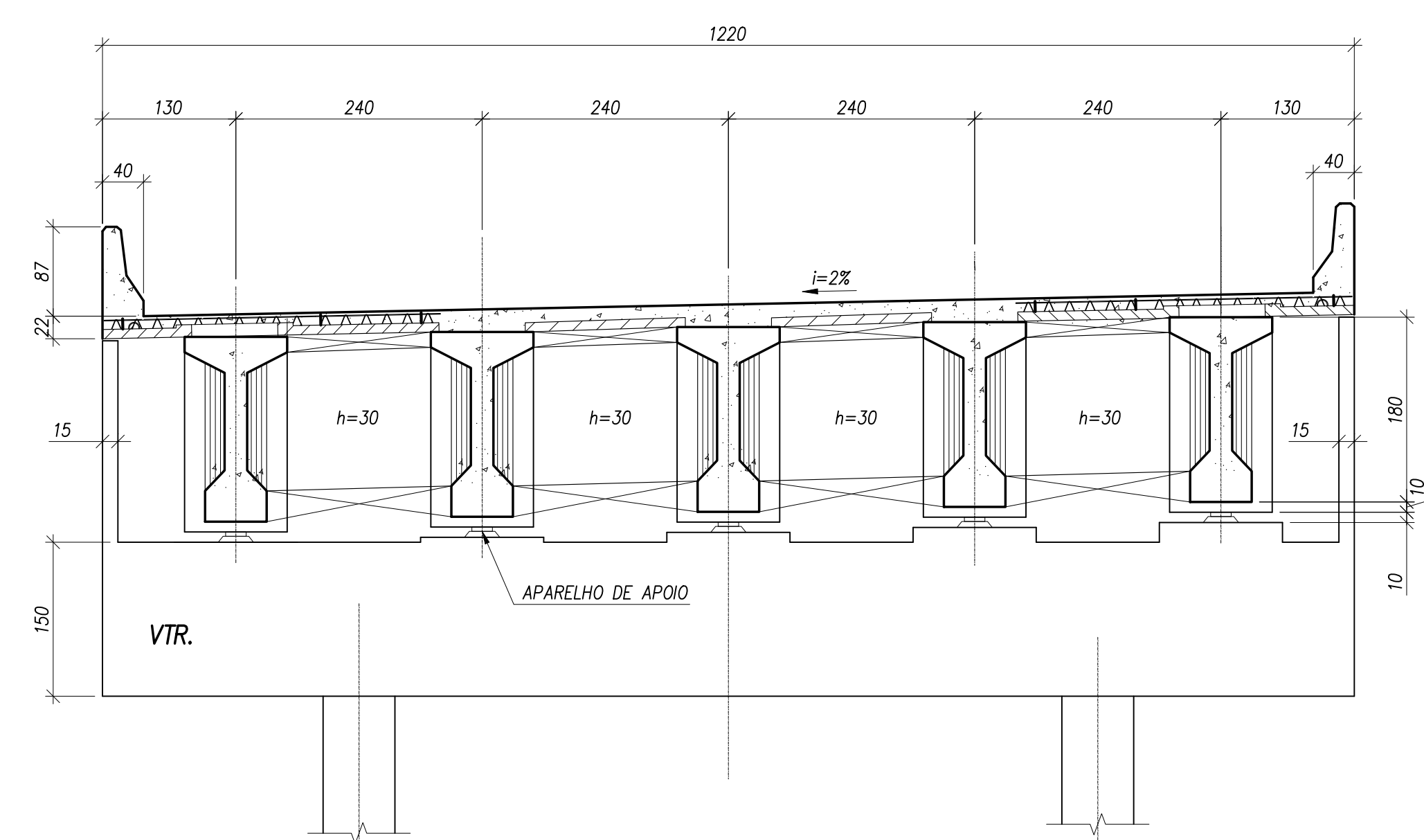
SEÇÃO TRANSVERSAL - ENCONTRO ESCALA 1:50
