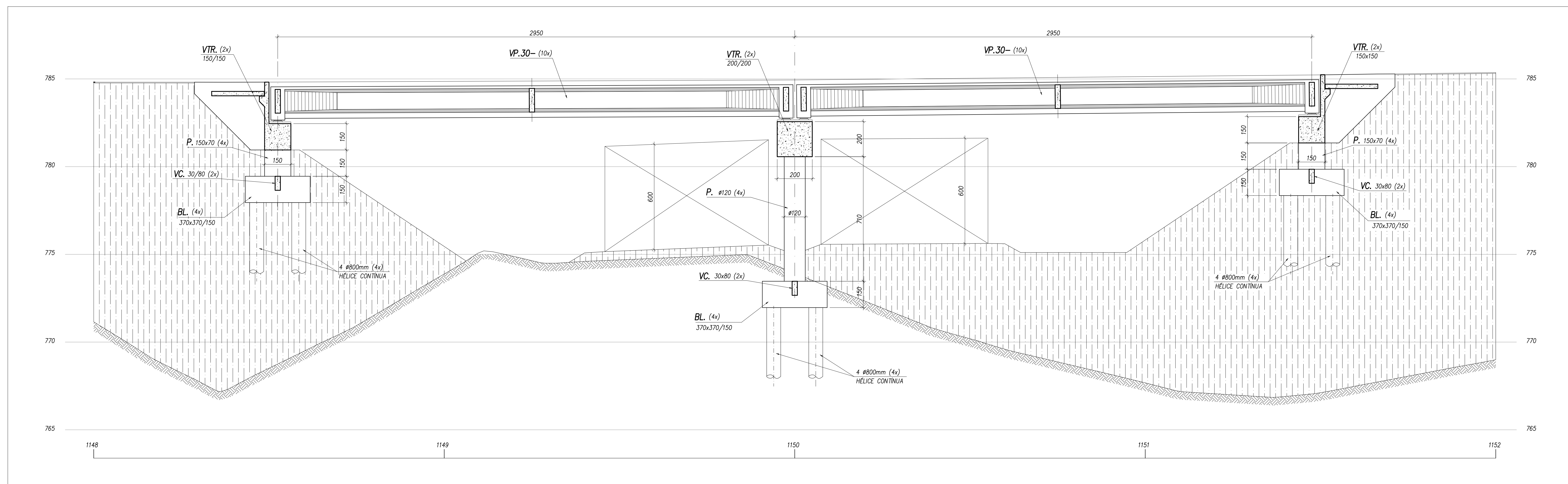
SEÇÃO LONGITUDINAL ESCALA 1:100
