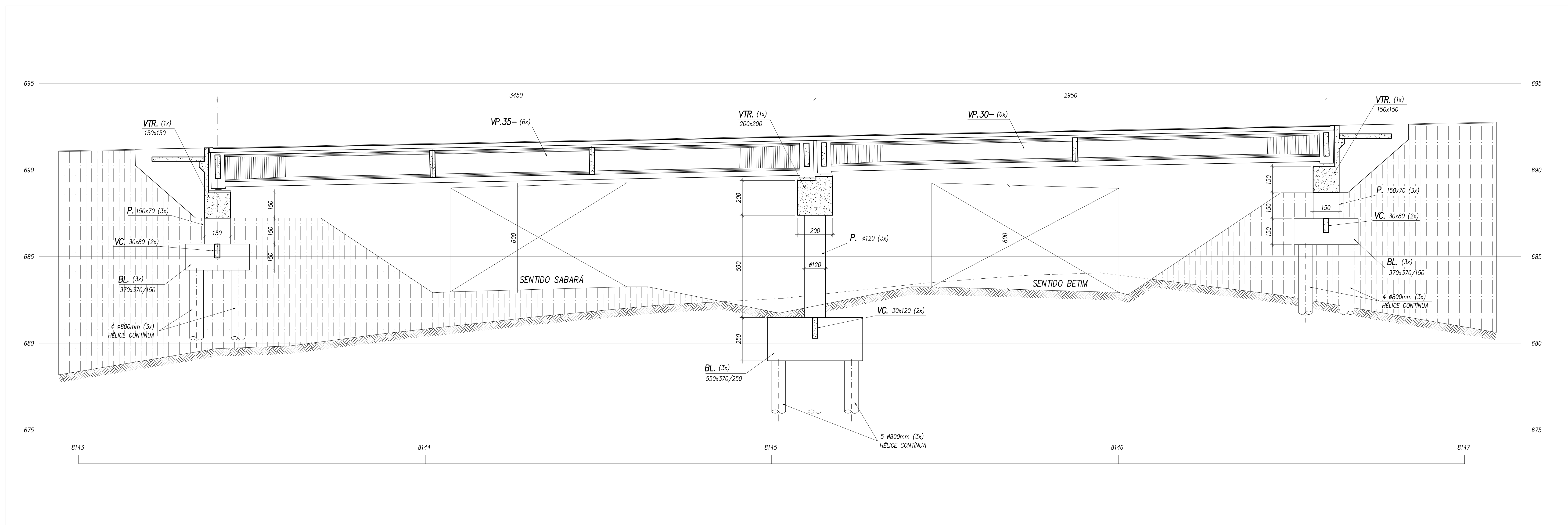
SEÇÃO LONGITUDINAL ESCALA 1:100
