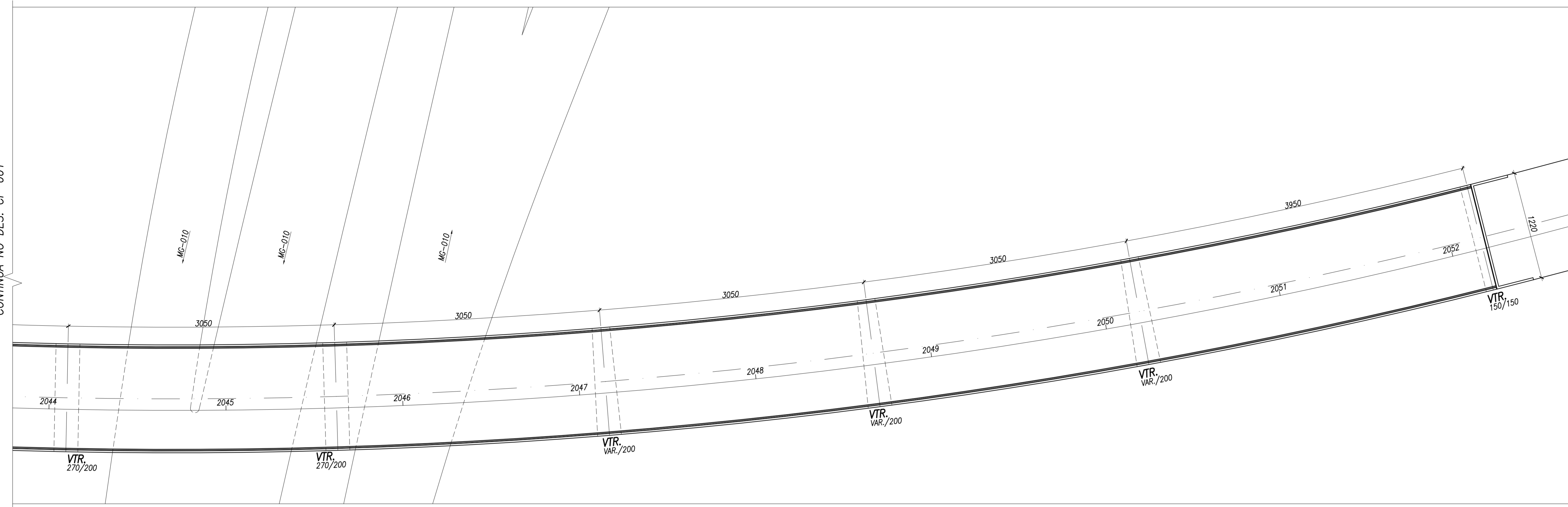
SUPERESTRUTURA - PLANTA ESCALA 1:250
