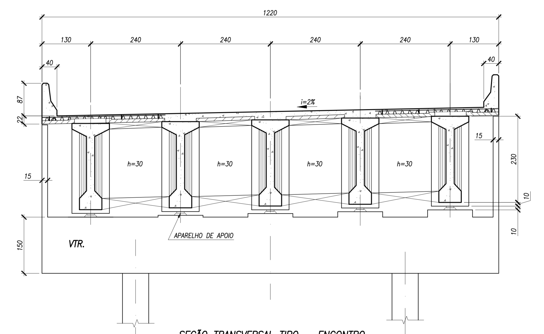
SEÇÃO TRANSVERSAL TIPO - ENCONTRO ESCALA 1:50
