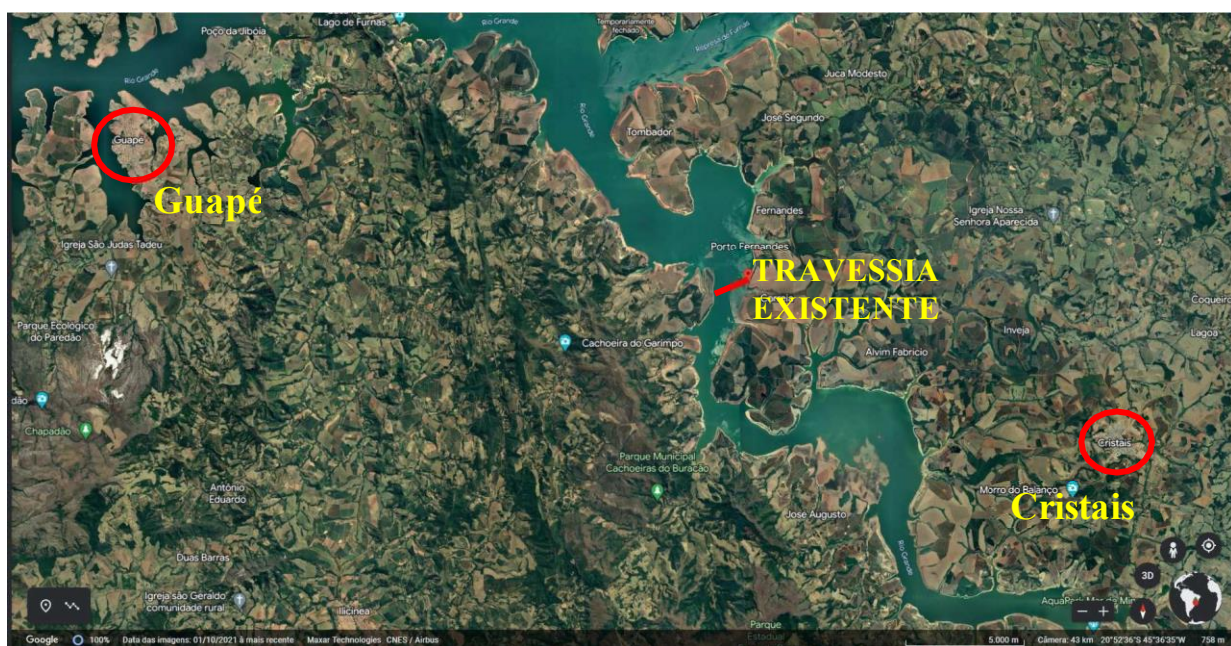
3.5-1 – UHE Furnas – Porto Fernandes - Vista de situação
