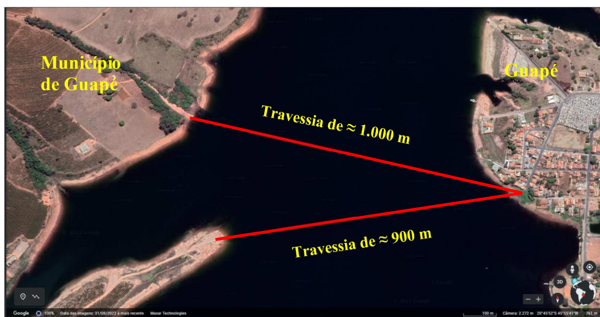
3.4-2 – UHE Furnas – Porto Barreirinho - Vista da Travessia existente
