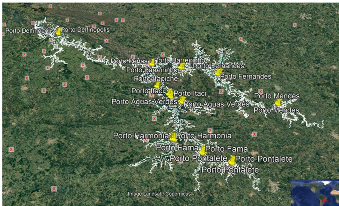
Foto 5-1 – Levantamento Topográfico dos Reservatórios da UHE Furnas e Mascarenhas de Moraes – Vista Geral
