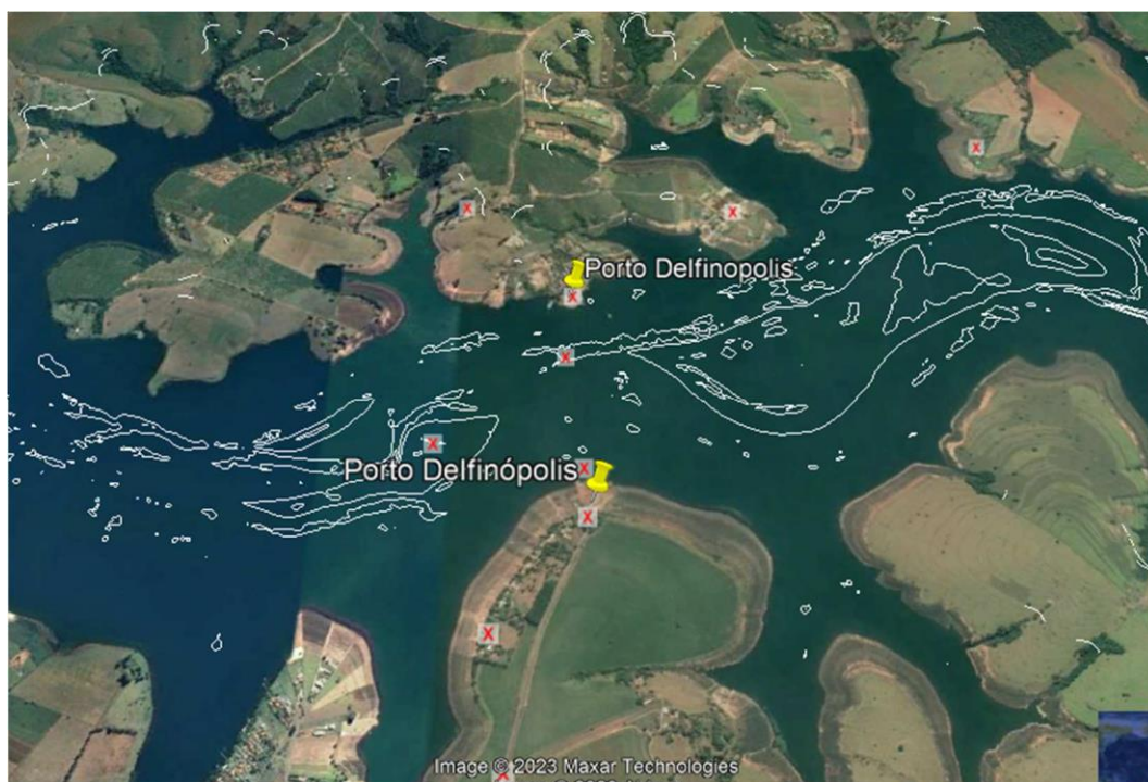
Foto 5-3 – Levantamento Topográfico dos Reservatórios da UHE Mascarenhas de Moraes – Porto Delfinópolis - Vista Geral
