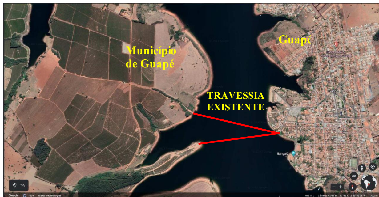
3.4-1 – UHE Furnas – Porto Barreirinho - Vista de situação
