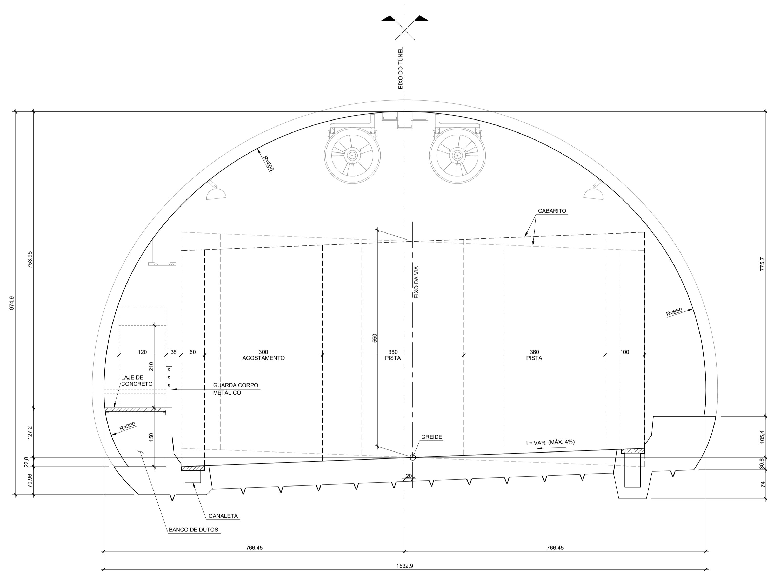
LEIAUTE - ELEMENTOS INTERNOS E GEOMETRIA ESC. 1:50
