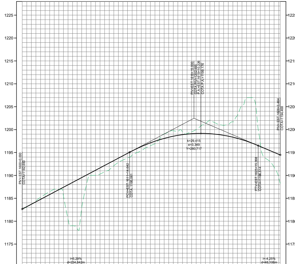
PERFIL RAMO 1600
