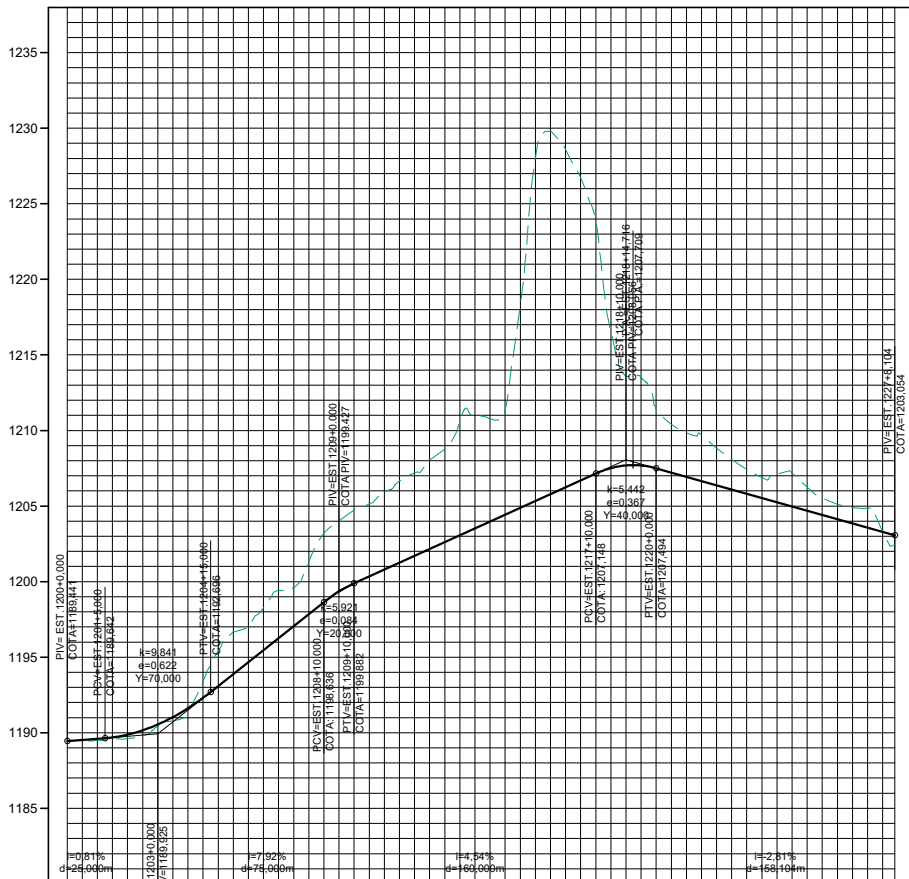
PERFIL RAMO 1200
