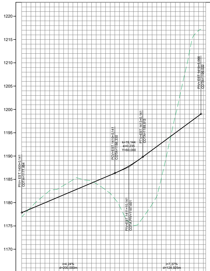
PERFIL RAMO 1400
