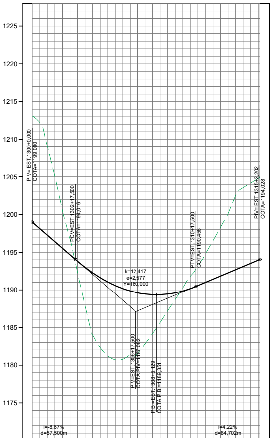
PERFIL RAMO 1300
