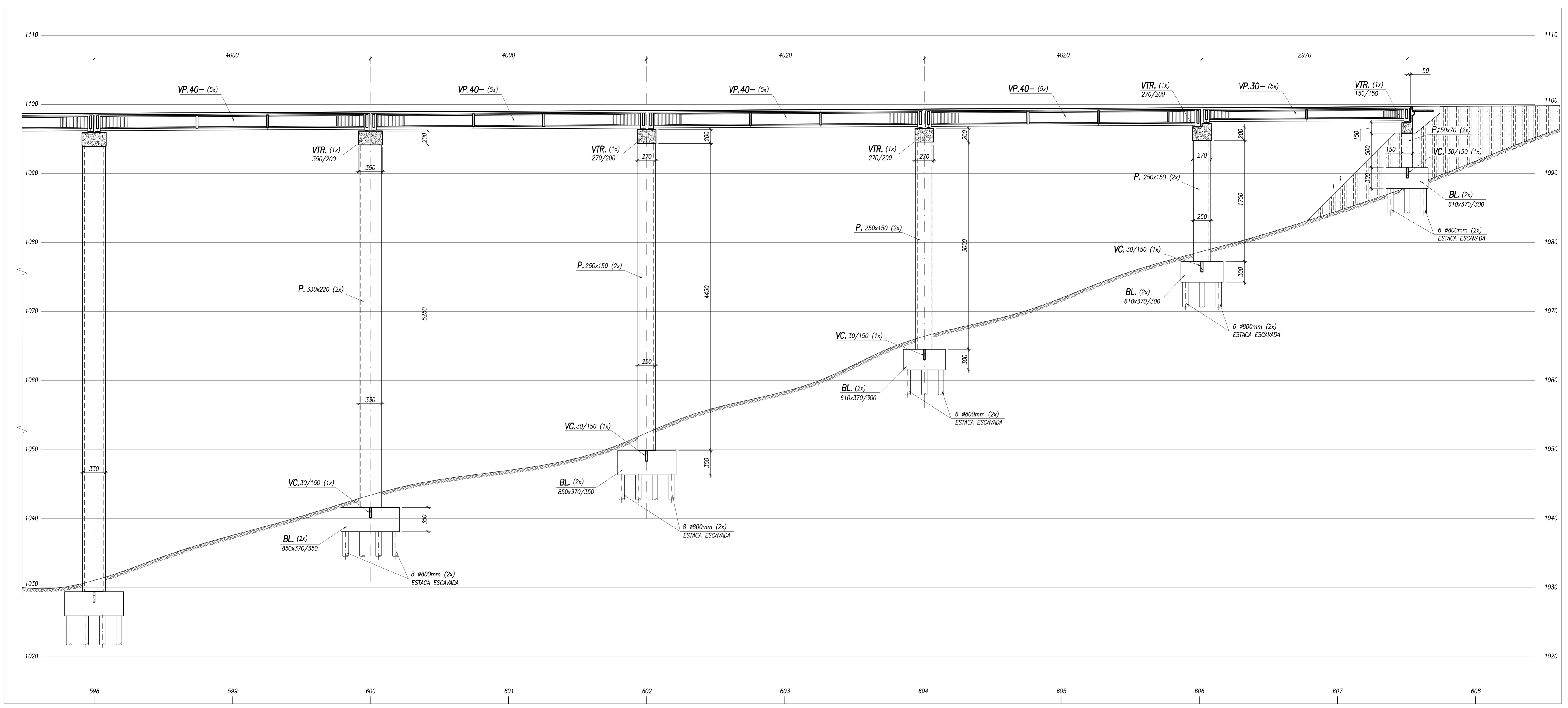
PERFIL LONGITUDINAL - 2a. PARTE ESCALA 1:250
