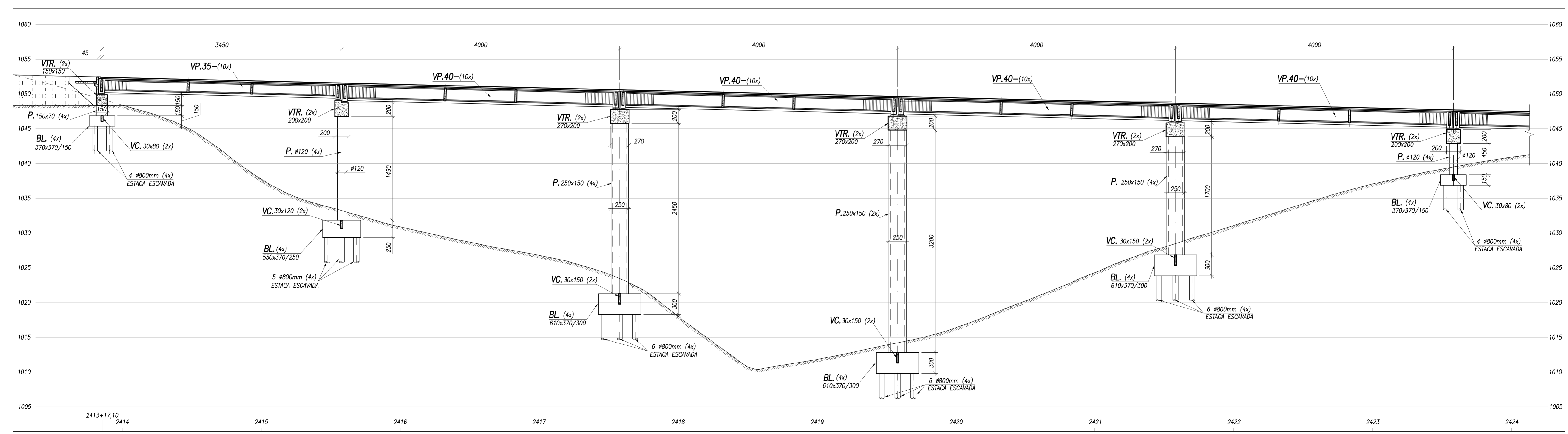
SEÇÃO LONGITUDINAL - 1ª PARTE ESCALA 1:250
