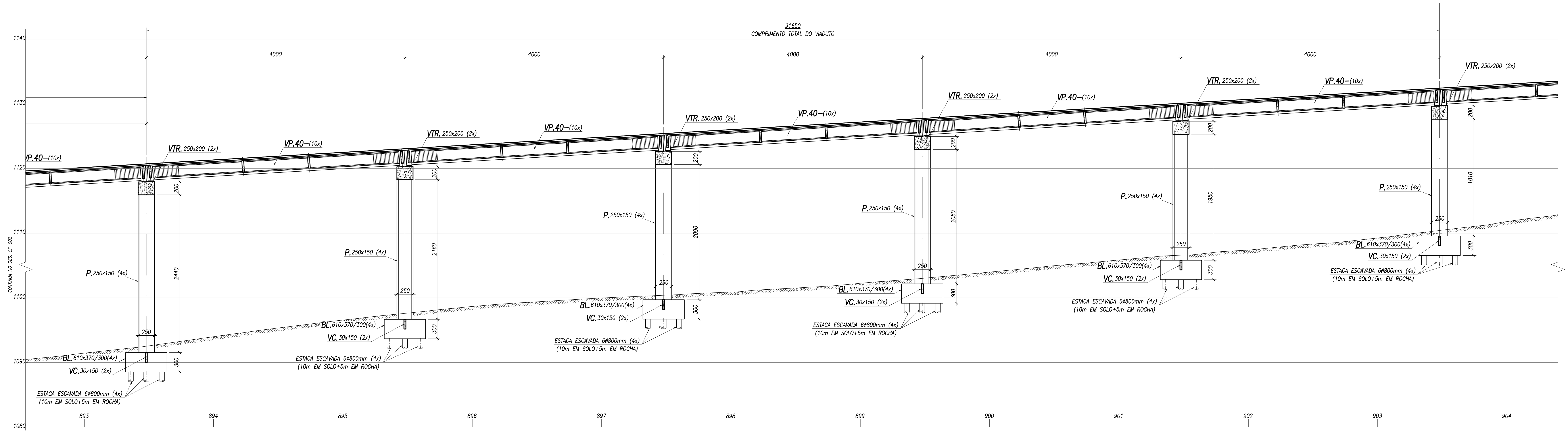
SEÇÃO LONGITUDINAL ESCALA 1:250
